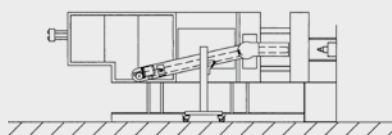
Posizione del nastro parallelo alla pressa. Parallel position of the conveyor respect the moulding machine.
