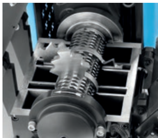
Cutting chamber view. Vista della camera di taglio.
