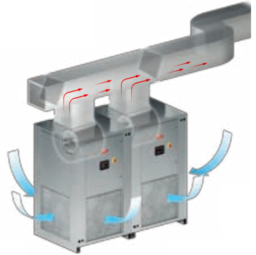
Functional scheme. Schema di funzionamento.
