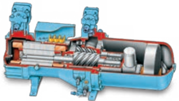
Screw compressor. Compressore a vite.
