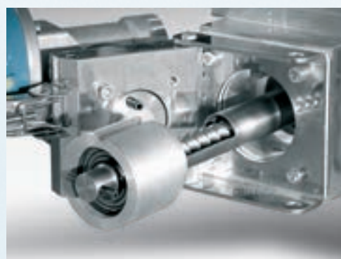
Extraction system of dosing screws. Sistema di estrazione rapida delle viti di dosaggio.
